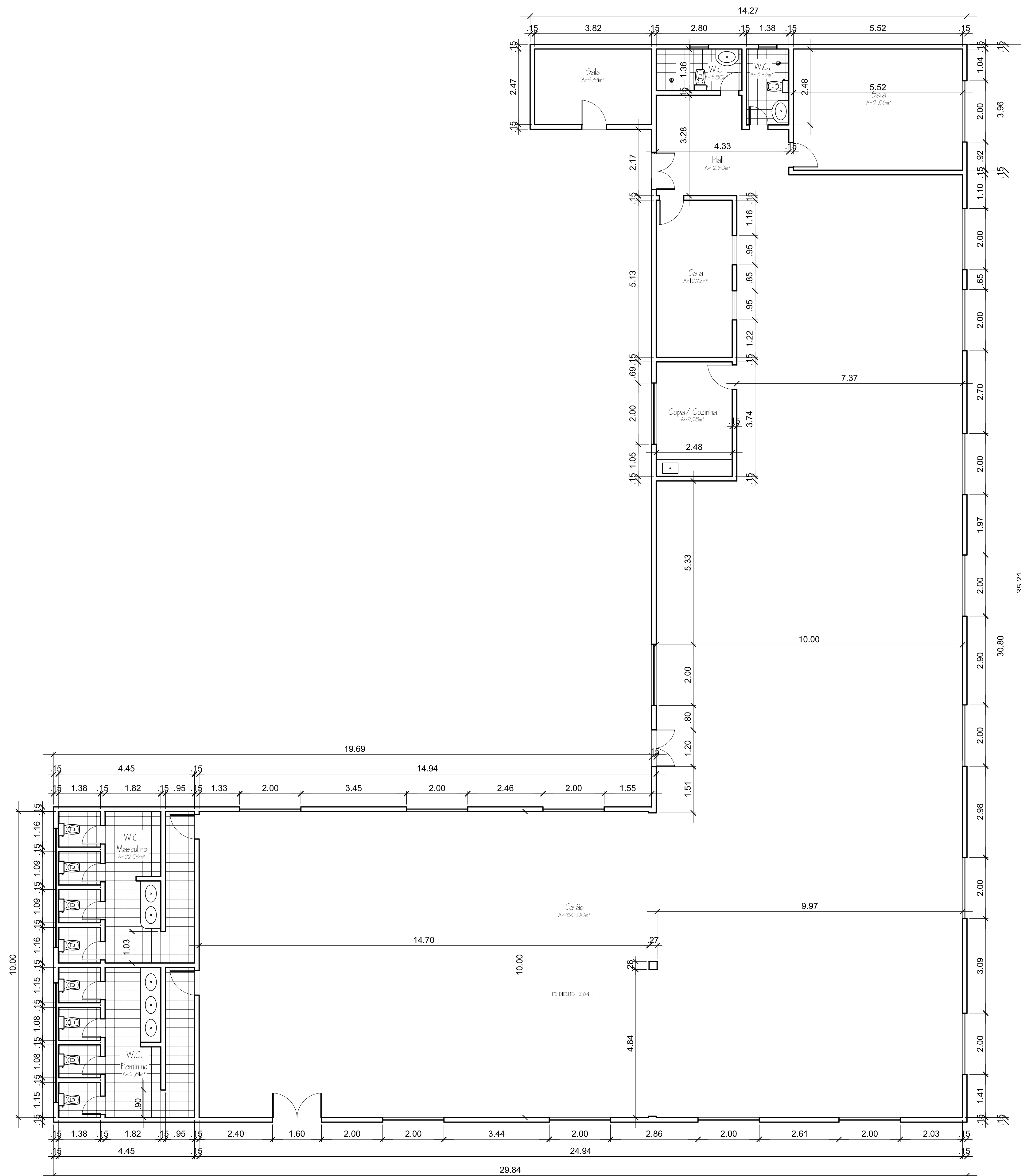
PLANTA BAIXA ESC. 1/75
